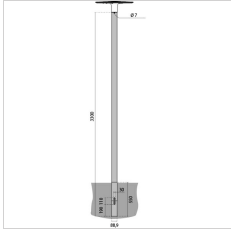
315023 Pole Spillo INT. 3.3 m
